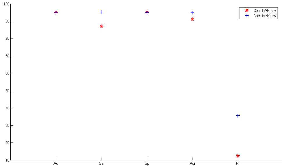
Figura 19: Gráfico - Avaliação da metodologia de inclusão de conhecimento adquirido para o organismo Rattus norvegicus . Apresenta os resultados obtidos com a metodologia de inclusão de conhecimento adquirido. Percebe-se que há um aumento de 22,09% na taxa de precisão ao se utilizar a metodologia proposta. Estes resultados foram obtidos utilizando-se o método de balanceamento M-Clus, e as características ATG + STOP + GAG.
