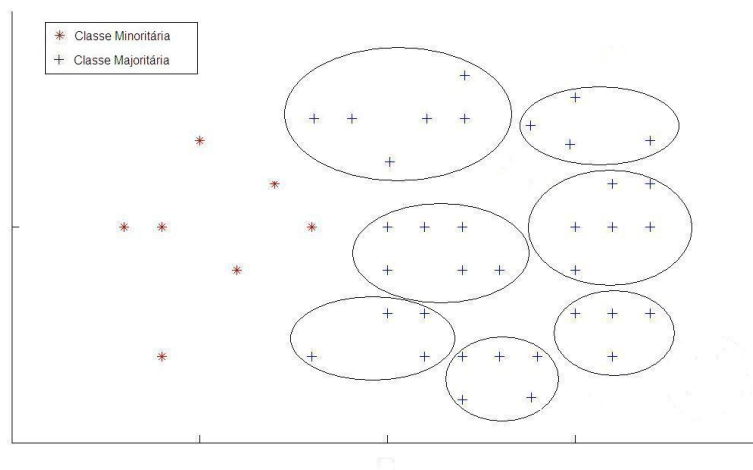
Figura 7: Funcionamento do método M-Clus. Os exemplos da classe majoritária são divididos em k clusters, onde k é a quantidade de elementos da classe minoritária. Posteriormente, são selecionados um exemplo por cluster, igualando, assim, a quantidade de elementos das classes majoritária e minoritária.
