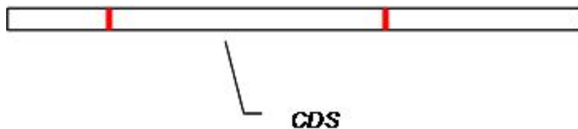
Figura 1: Exemplo de região codificadora (CDS).
